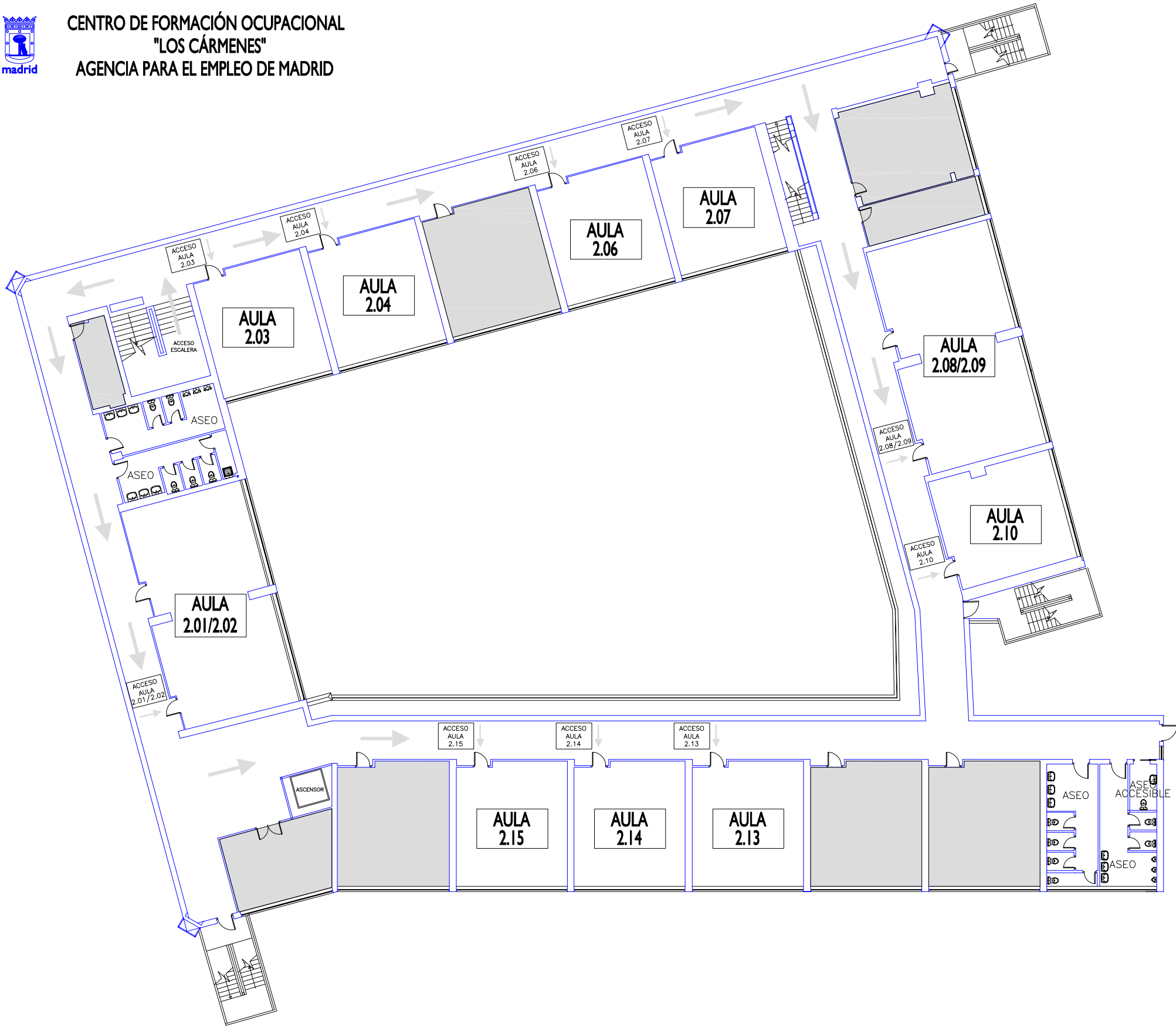
PLANTA DE AULAS. SEGUNDO EJERCICIO OPOSICIÓN ARQUITECTURA TÉCNICA 18/10/2025 (PLANTA SEGUNDA)
