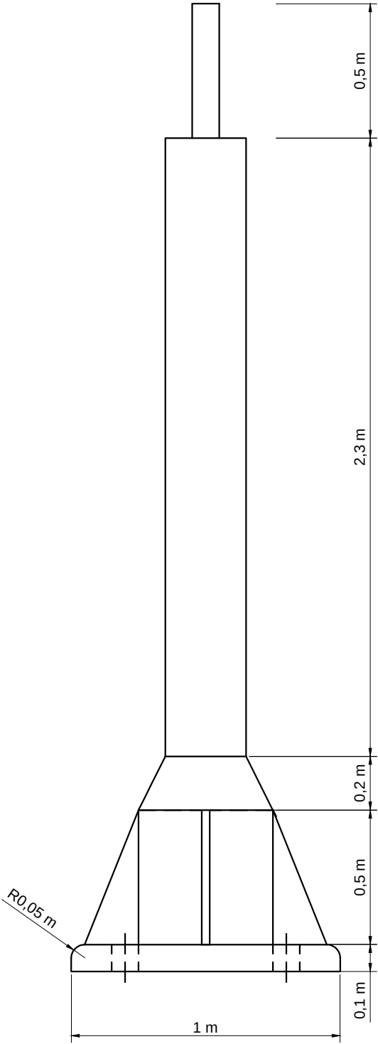
ALZADO
