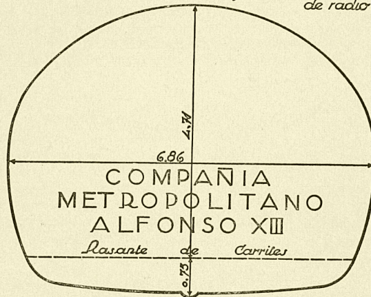
Sección de galería - En recta y curva hasta 200m. de radio.
