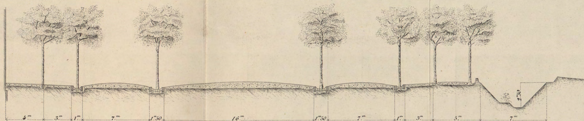
Perfil trasversal del Camino ó Paseo de ronda y foso de circuito
