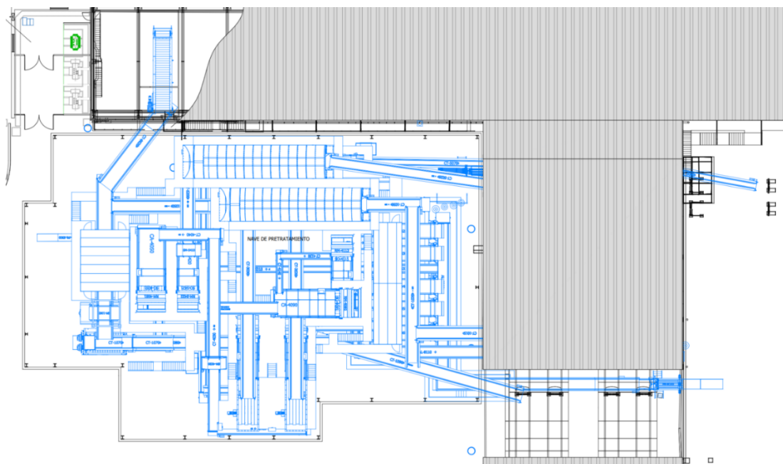
Plano de la planta de separación y clasificación de Las Lomas
