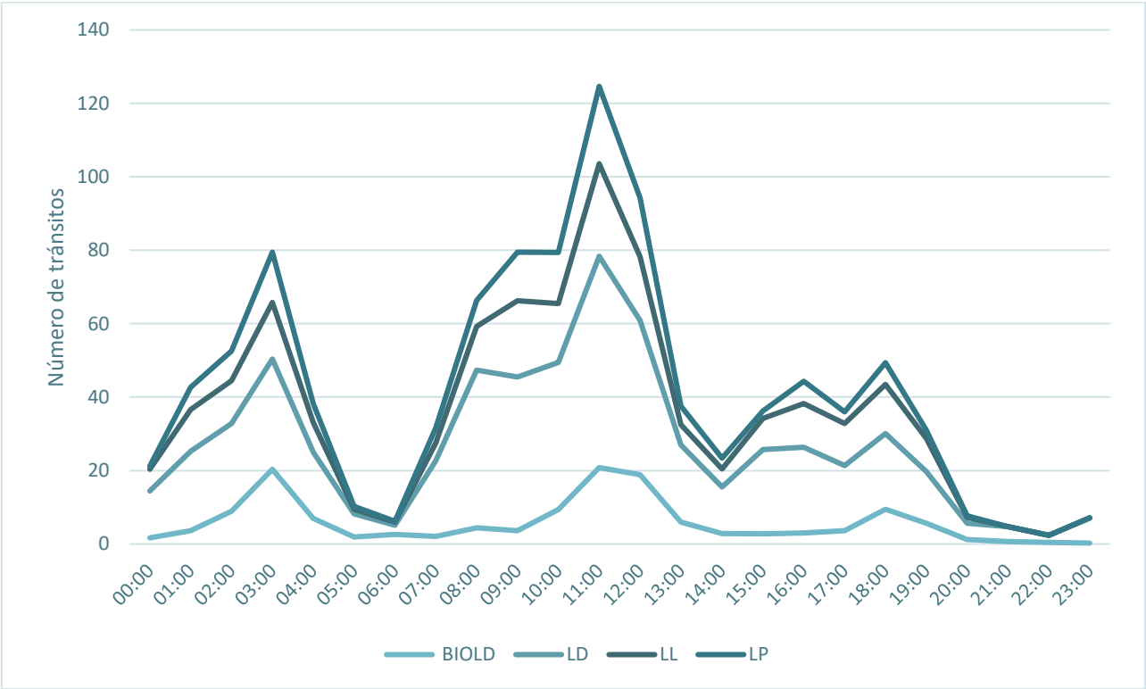
Gráfico 2.9. Distribución horaria de los camiones que acceden al PTV, por planta (2023)
