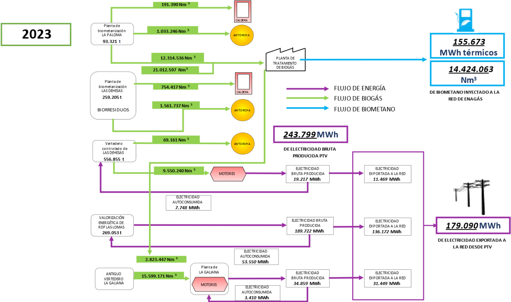
Gráfico 1.12. Principales flujos de biogás y energía del PTV (2023)
