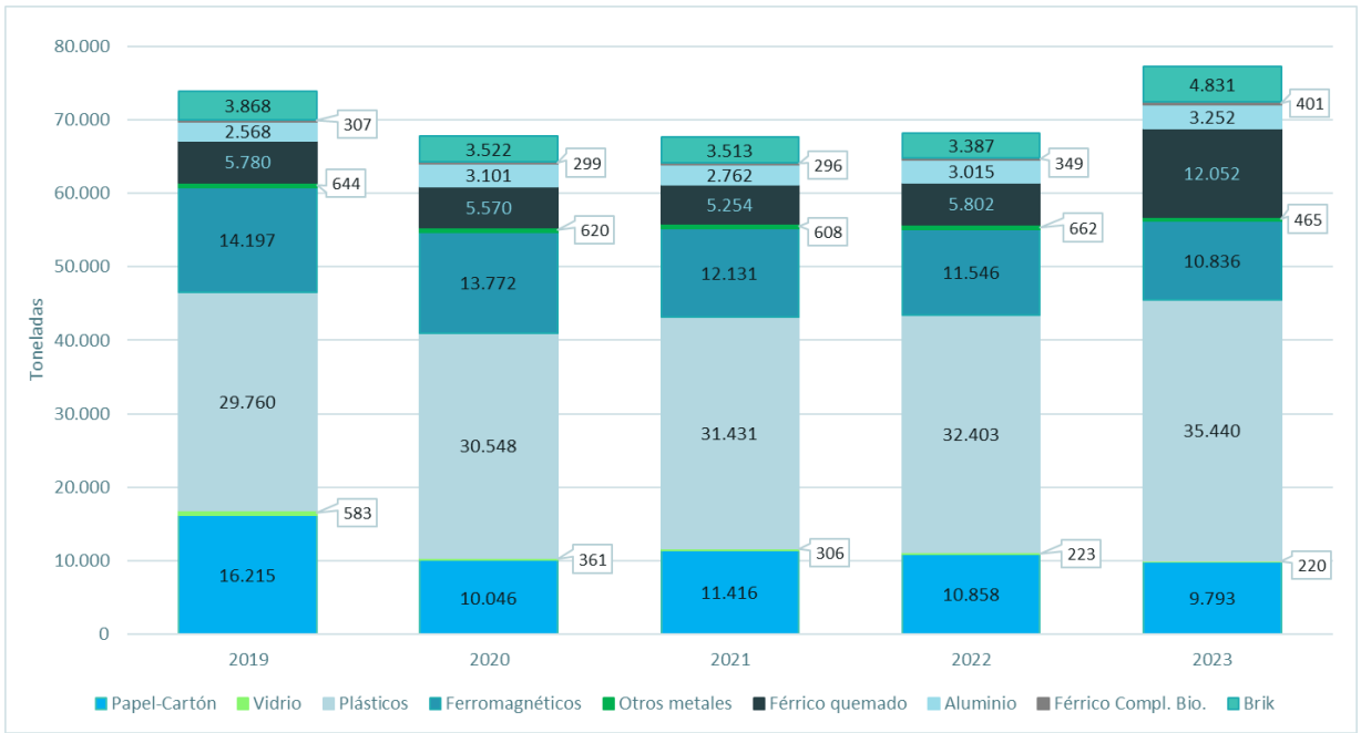
Gráfico 1.8. Materiales recuperados en el PTV de 2019 a 2023, en toneladas
