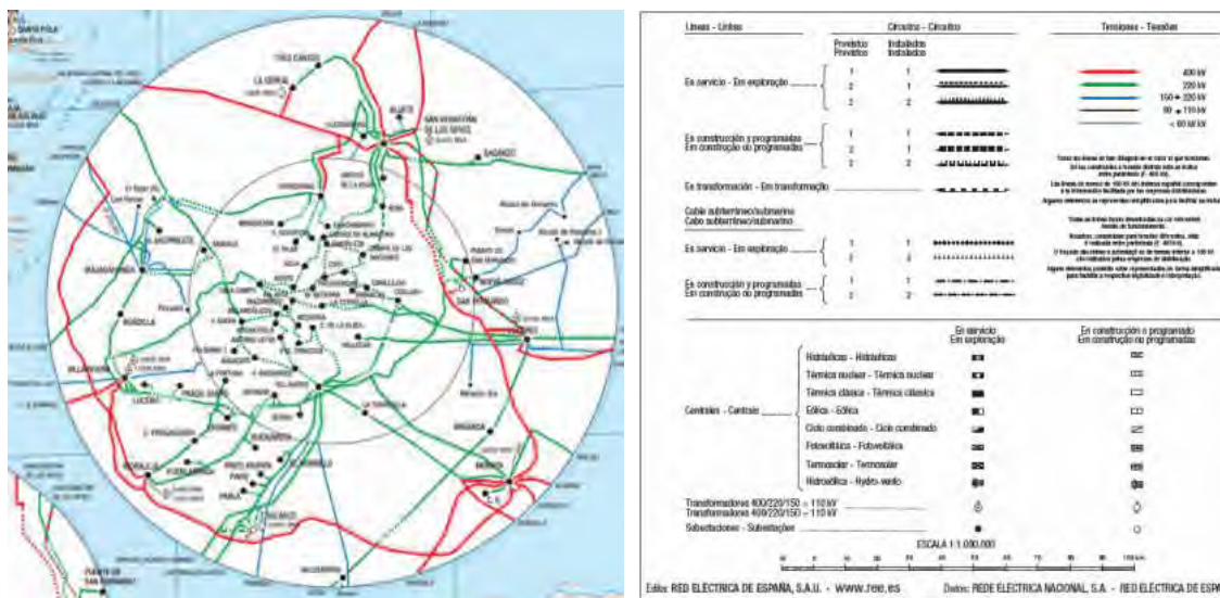
Fig. 49 Mapa del Sistema Eléctrico Madrid
