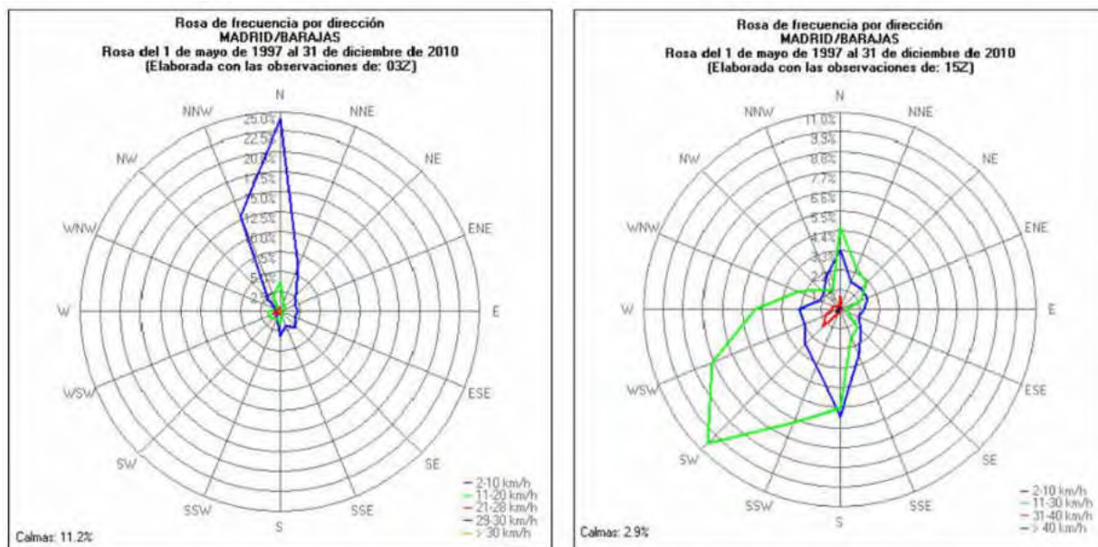
Fig. 21 Rosa vientos Madrid / Barajas (LEMD)
