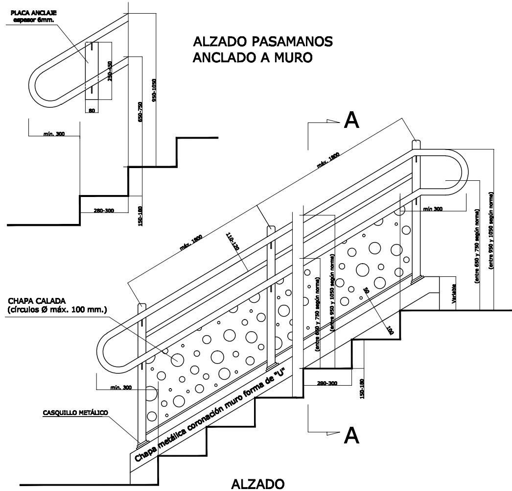
DETALLE TIPO BARANDILLA-PASAMANOS ESCALERA
