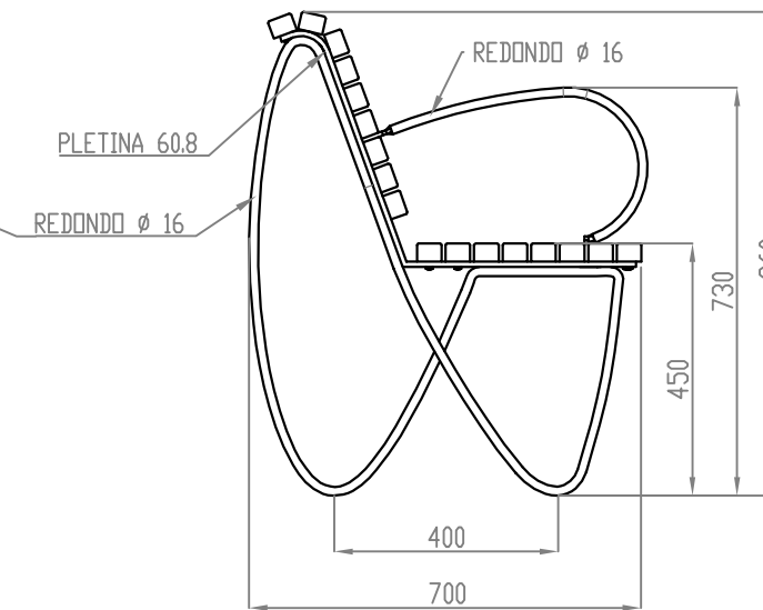
ALZADO LATERAL
