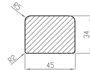
SECCIÓN LISTON ESCALA 1:2
