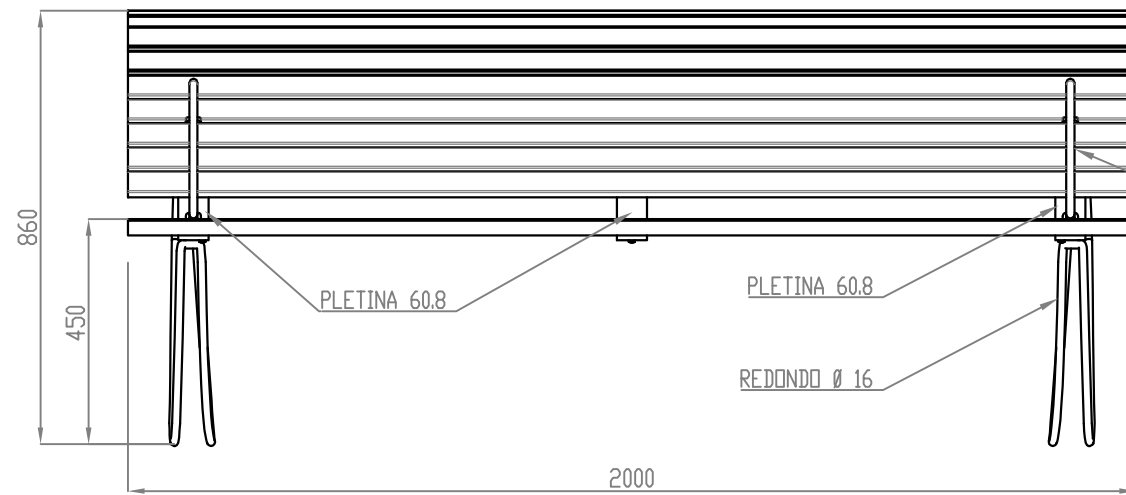
ALZADO FRONTAL
