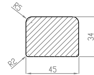
SECCIÓN LISTON ESCALA 1:2
