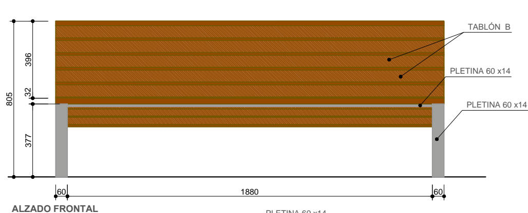
ALZADO FRONTAL
