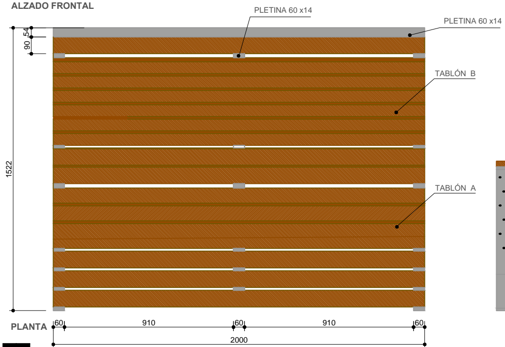
ALZADO FRONTAL
