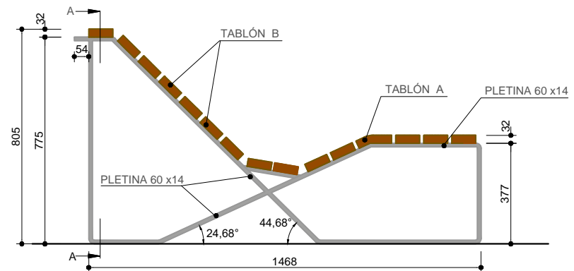
ALZADO LATERAL
