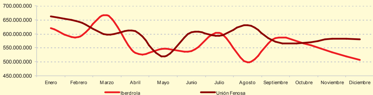
Electricidad facturada (kWh) en la Ciudad de Madrid por meses. Año 2006
