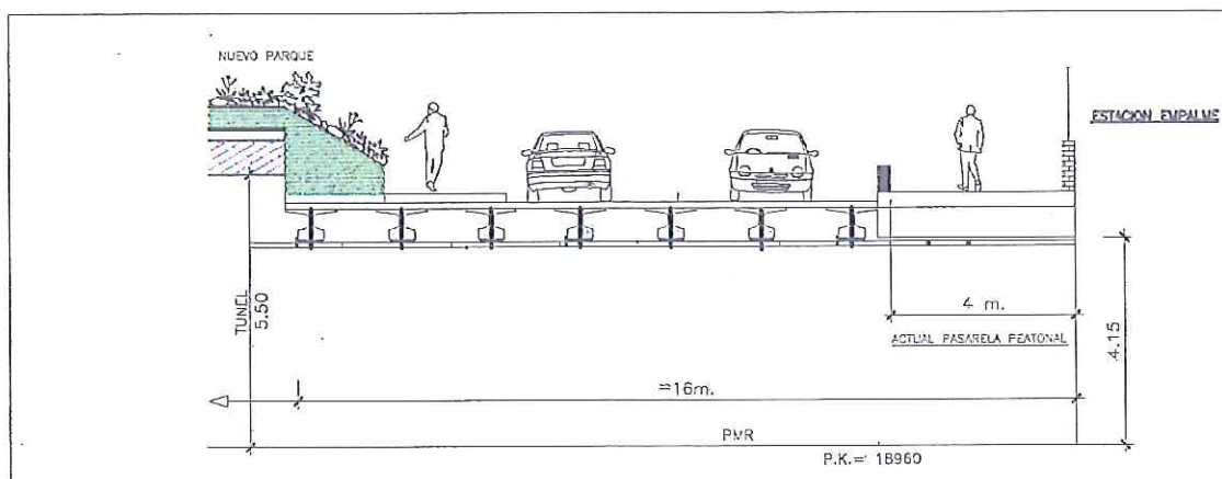
Detalle bajo calzada prolongación calle Tembleque
