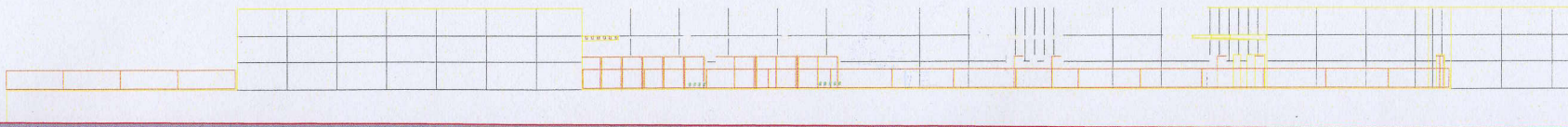
Alzado sur
