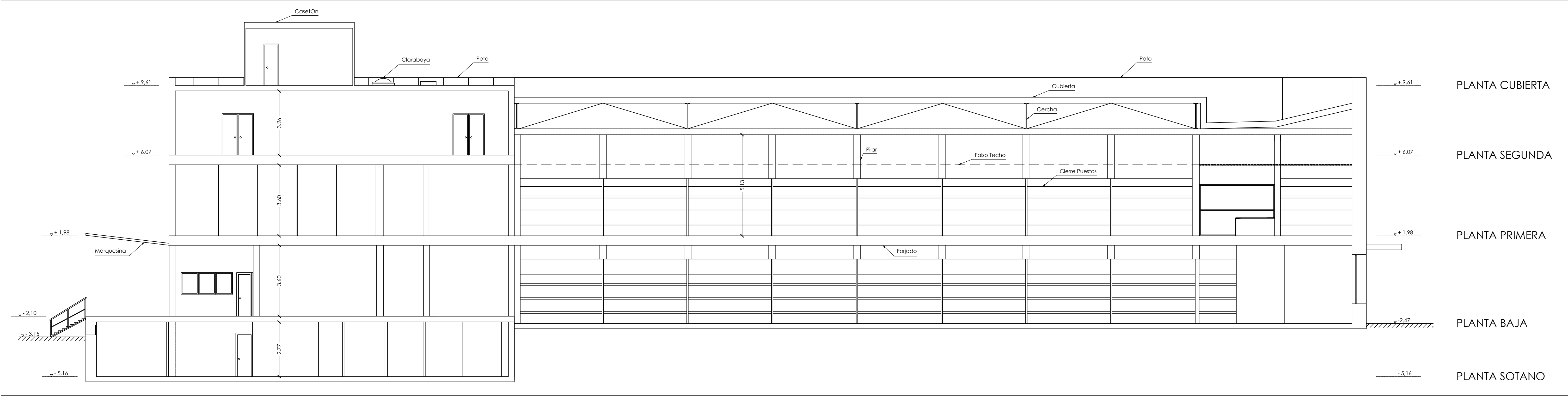
SECCIÓN A-A'
